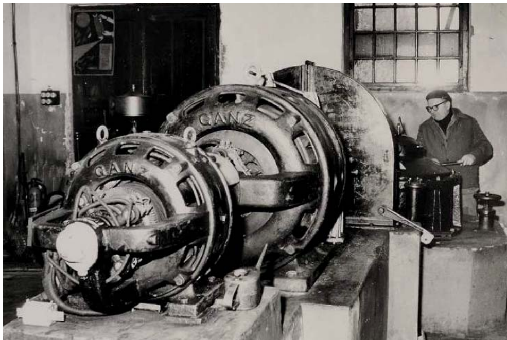
Turbina-generátor a villanytelepen
