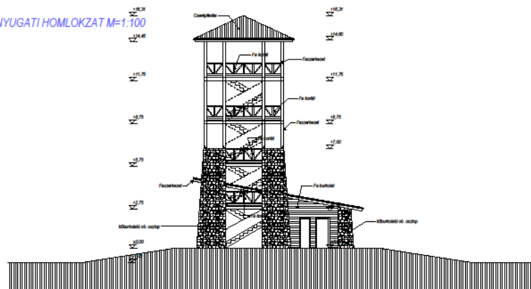
ÉSZAKI HOMLOKZAT M=1:100
